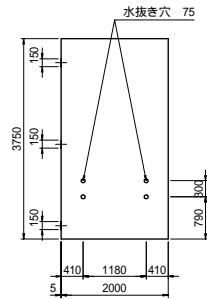
正面形状図
