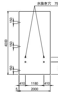
正面形状図
