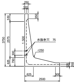
断面形状図
