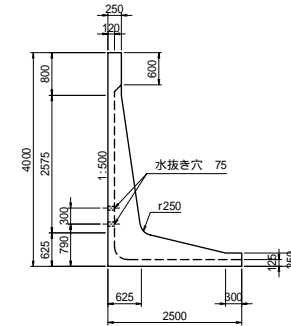
断面形状図
