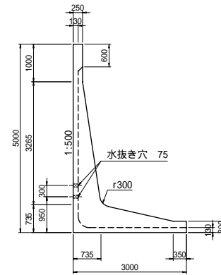
断面形状図
