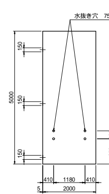
正面形状図
