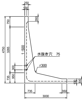
断面形状図
