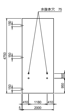
正面形状図
