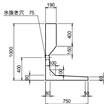
断面形状図
