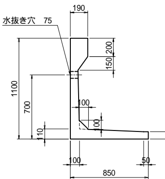
断面形状図
