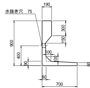
断面形状図
