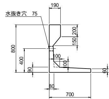
断面形状図
