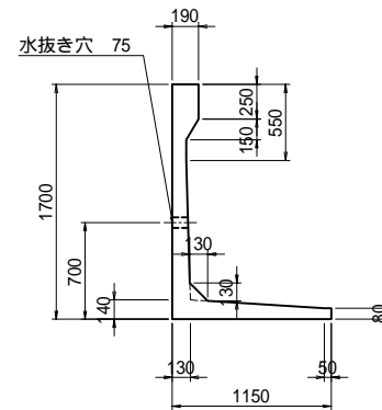
断面形状図
