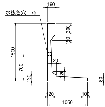
断面形状図
