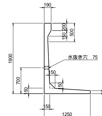
断面形状図
