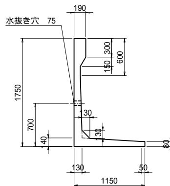
断面形状図
